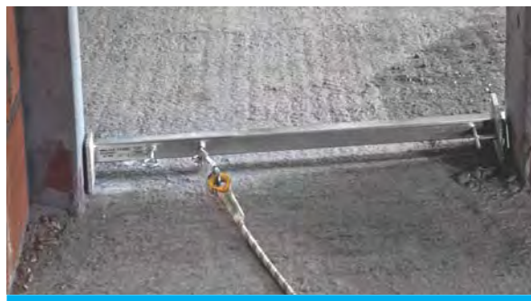
Kotwienie do belki poprzecznej mocowanej w otworach ściennych.
