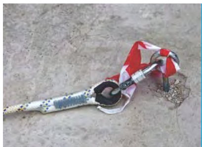
Kotew punktowa mocowana w betonie.
